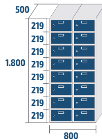
ECOZ-40/2 COD: 84822 56,8kg · 0,72m 3
