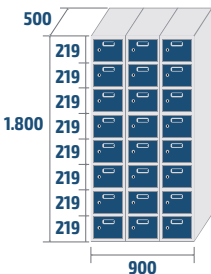
ECOZ-30/3 COD: 83823 70,1kg · 0,81m 3
