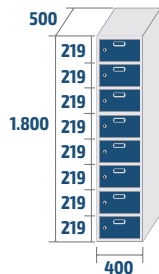
ECOZ-40/1 COD: 84821 30,9kg · 0,36m 3
