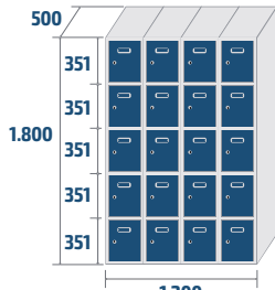
ECOP-30/4 COD: 83064 75,9kg · 1,08m 3
